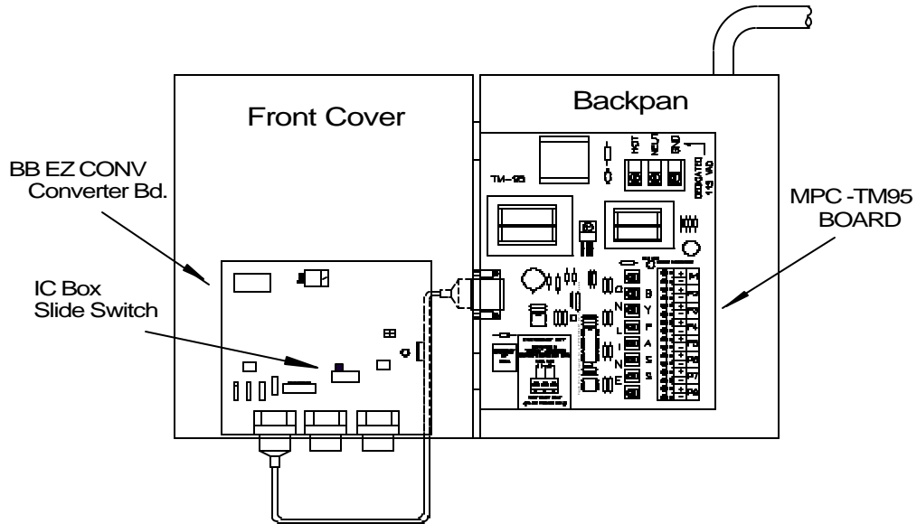
Fig. 7, PetroSmart EZ, Cat IC Box
